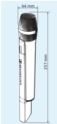
Maße SKM 5200
